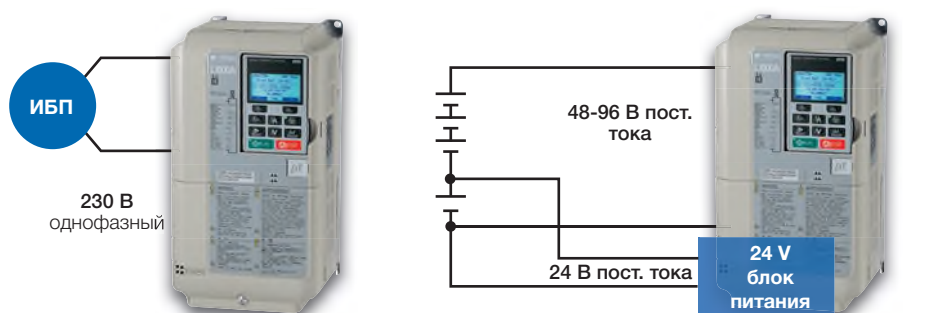
Проводка и эксплуатация ИБП Проводка и эксплуатация резервной батареи
