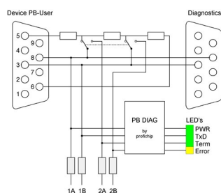
Wiring diagramm - Connector 90°
